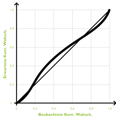
Abbildung 36: P-P Plot
